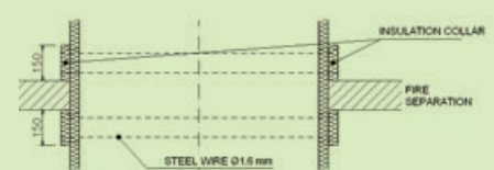
Tűz megállítási kör keresztmetszetű vezeték esetén
