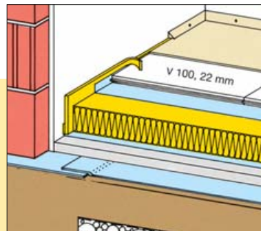
3 Fa építőlemez száraz burkolat *kétrétegű, ragasztott, csavarozott ISOVER TDPT 60/60
