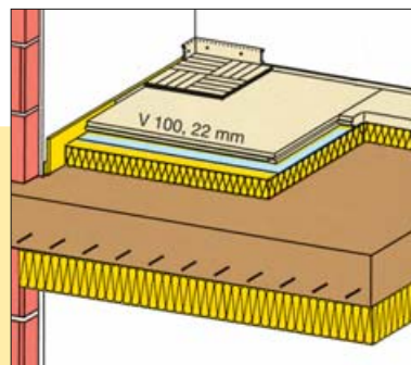
3 Száraz burkolat: ISOVER TDPT 50/50, 6 cm ISOVER KDP vagy 12 cm ISOVER KDP
