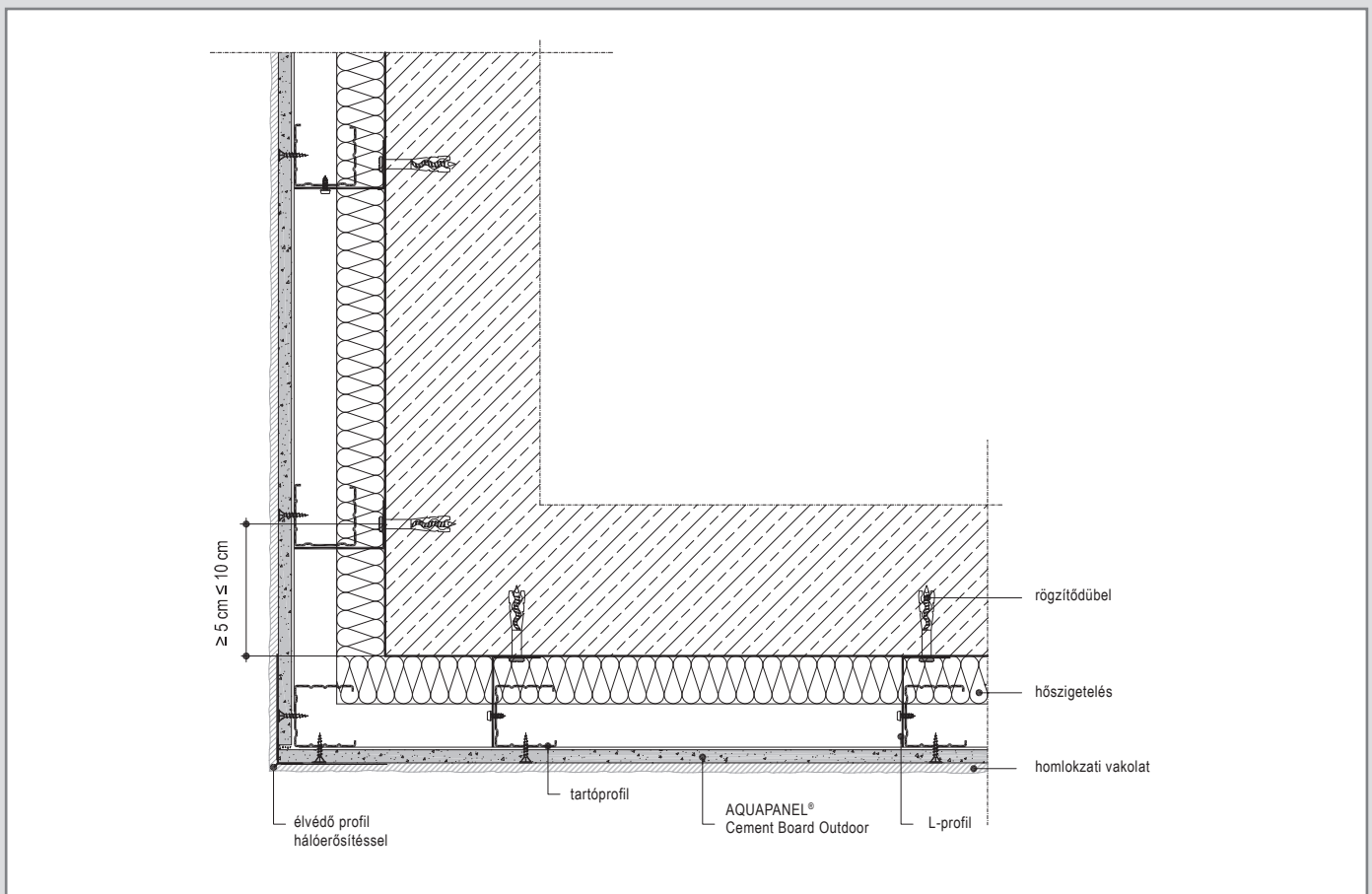
W682-E1 Pozitív sarok
