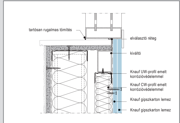
W388E-FE-VU2 Párkány kialakítás 2
