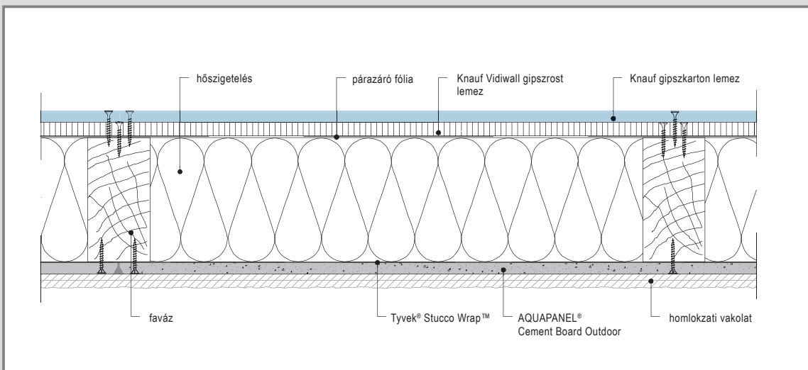
W571-H1 Alaprajzi kialakítás
