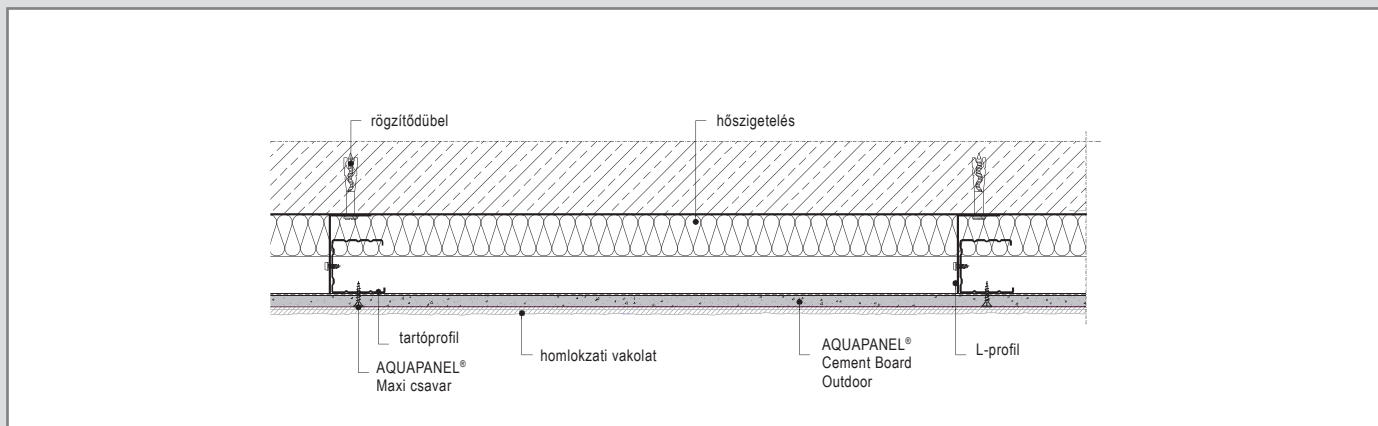
W682-H1 Alaprajzi kialakítás
