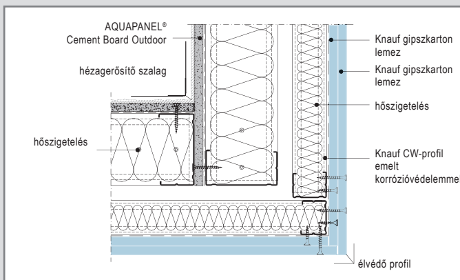
W388E-D1 Negatív sarok kialakítás
