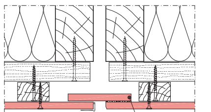
Vidiwall lemezcsík Vidiwall Fillerrel vagy Uniflittal az egyik oldalhoz ragasztva
